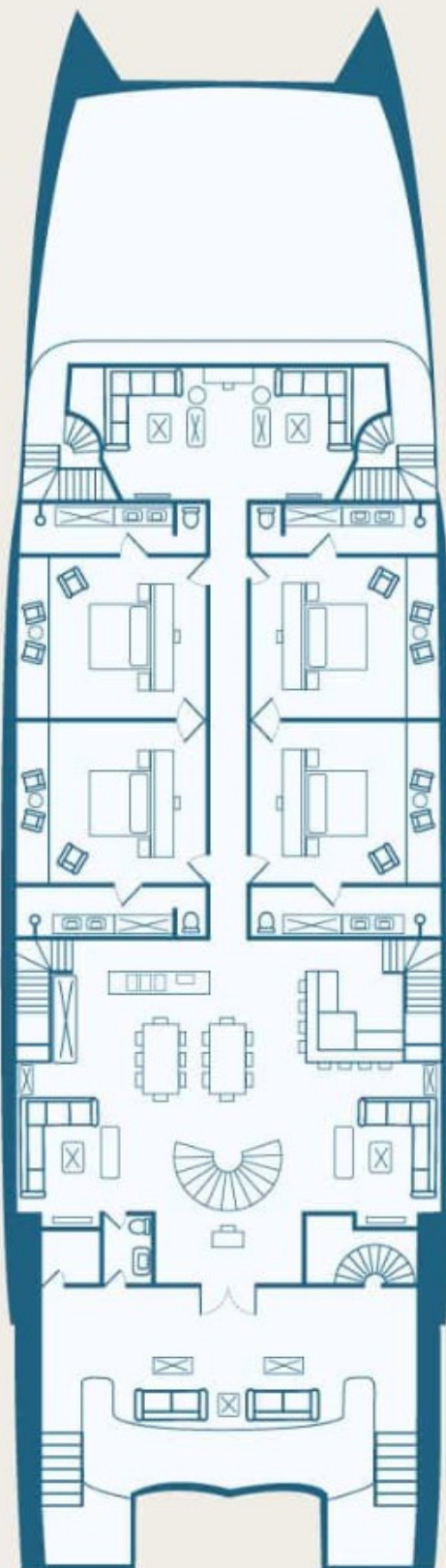
Hauptdeck
